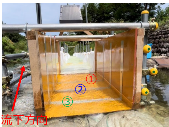
誘導水路内壁に電極を3つ設置
